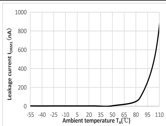
图 10 抑制电压 vs 环境温度
