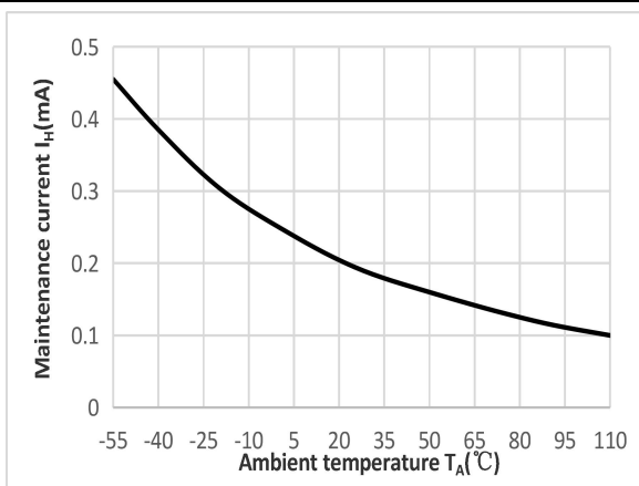
图 9 抑制状态泄漏电流 vs 环境温度
