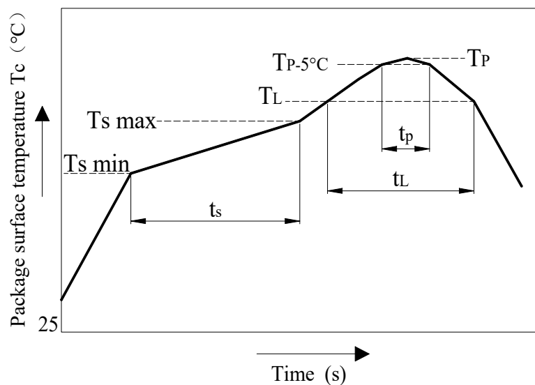
回流焊温度曲线图 Solder Reflow Profile
