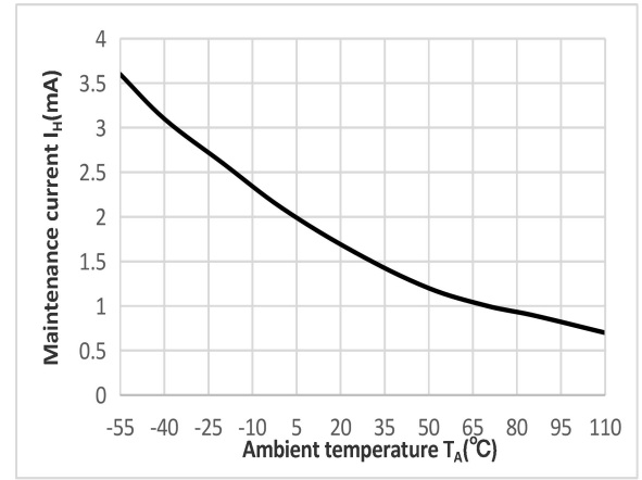
图8 抑制状态泄漏电流 vs 环境温度
