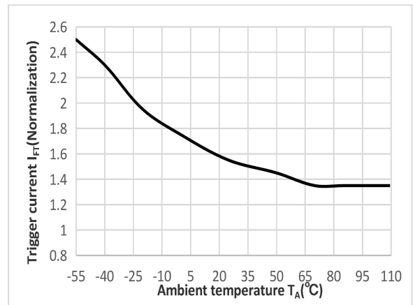
图6 维持电流 vs 环境温度
