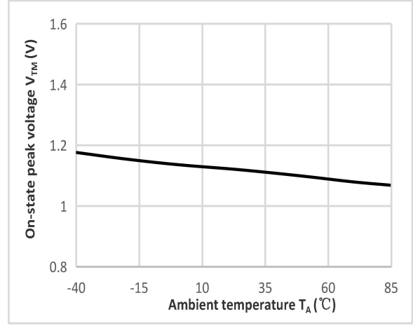
图 4 正向压降 vs 环境温度
